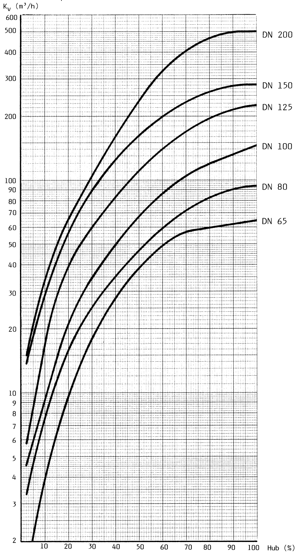
k_v - Werte in Abhängigkeit vom Hub
