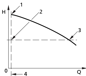
Q-H - Diagramme
