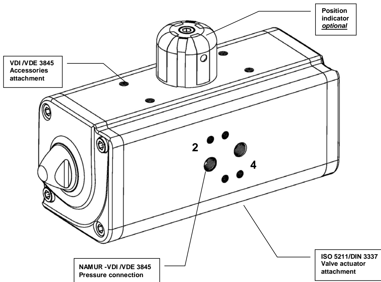
Fig 5,1 - Actuator control.
