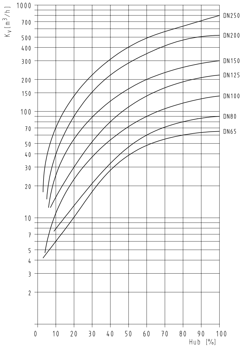
K_V -Werte in Abhängigkeit vom Hub
