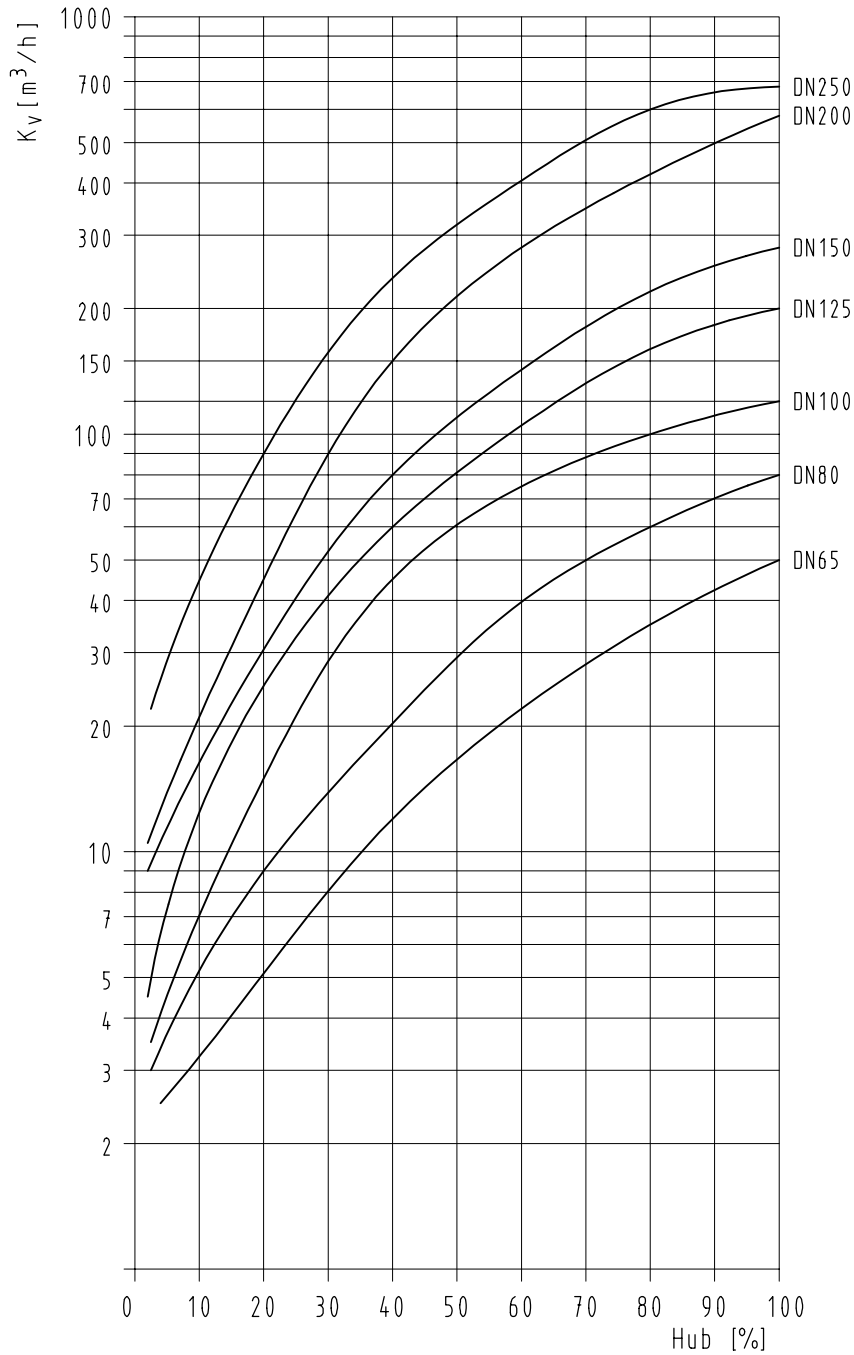
k_V - Werte in Abhängigkeit vom Hub
