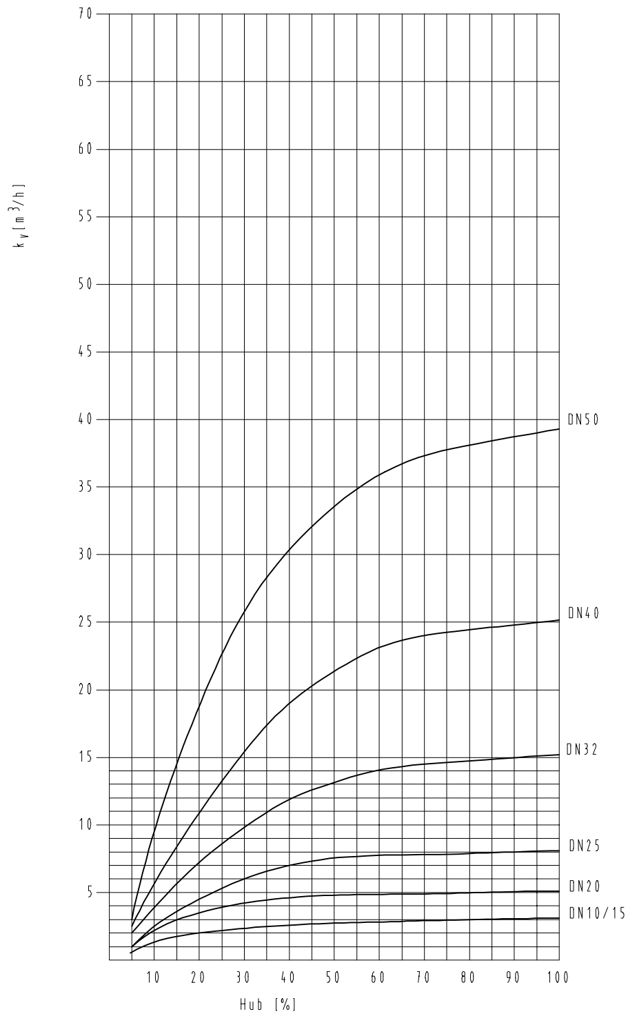
k_v - Werte in Abhängigkeit vom Hub
