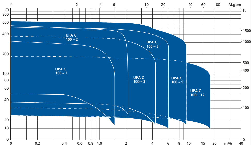
Kennlinien UPA C 100 CC (50 Hz)
